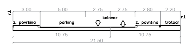
poprečni profil A - A
